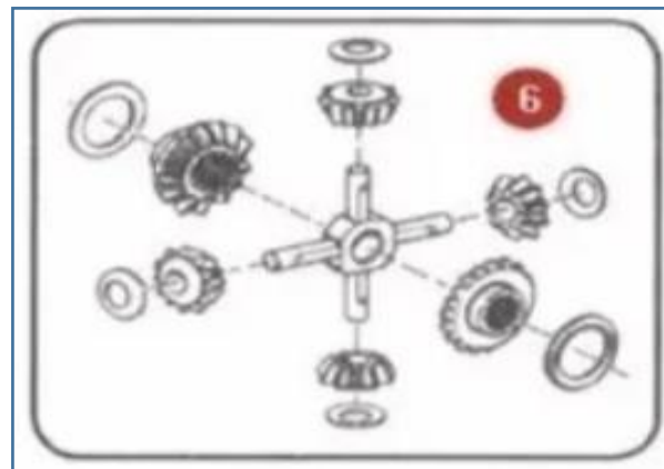
CONJUNTO DE BLOQUEIO DIFERENCIAL (CAIXA SATÉLITE) ILUSTRATIVO
