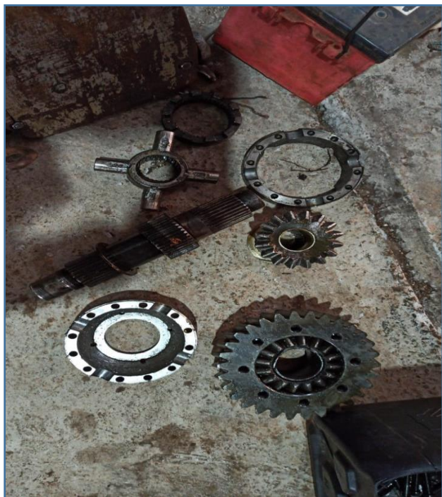
CONJUNTO DE BLOQUEIO DIFERENCIAL (CAIXA SATÉLITE) DESMONTADO / DANIFICADO
